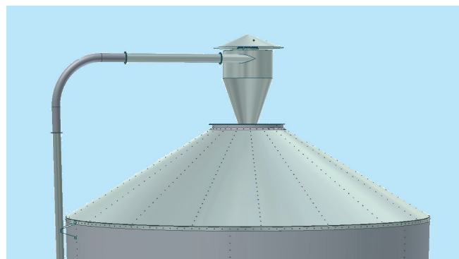
Unik XB-silo utrustad för torr lagring med inblåsningsrör och cyklon.
