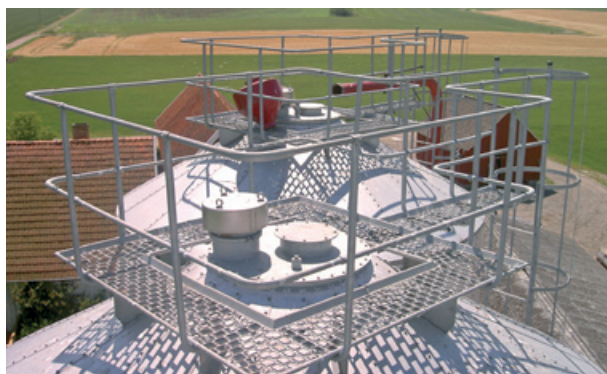
Takplattform med räcke samt över- och undertrycksventil för fuktig lagring samt cyklon (röd) för fyllning av silon.
