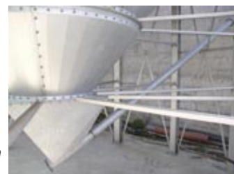
Kraftig afstivning af ben på siloen.
